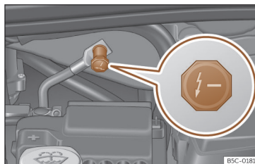
Abb. 175 Im Frontraum: Starthilfepunkt (Masseanschluss).
