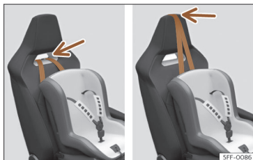
Abb. 42 Beifahrersitz: Einstellung und Einbau unter Verwendung des Top Tether-Gurts.
