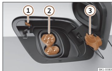
Abb. 58 Hinter der Batterieladeklappe hinten rechts: Ladedose.
