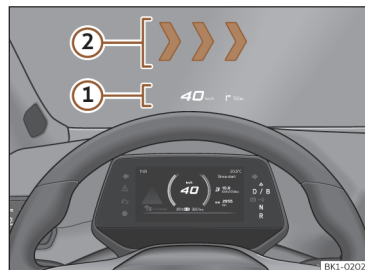
Abb. 4 Im Sichtfeld des Fahrers: HUD mit Annäherungsdaten ① und HUD mit AR ②.
