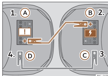
Abb. 176 Anschlussplan der Starthilfekabel.
