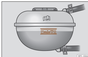
Abb. 185 Im Frontraum: Markierung am Kühlmittelausgleichsbehälter.
