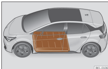
Abb. 52 Einbauort der Hochvoltbatterie
