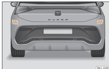
Abb. 112 Bereich hinter dem Fahrzeug: Bereiche der Radarsensoren.
