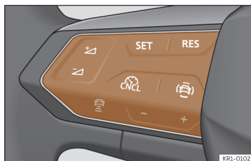
Abb. 115 Am Multifunktionslenkrad: Tasten zur Bedienung des Geschwindigkeitsbegrenzers.
