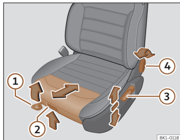
Abb. 84 Vordersitze: Manuelle Sitzverstellung.
