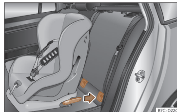
Abb. 38 Rückseite: Einbau des Kindersitzes mit dem ISOFIX-System.
