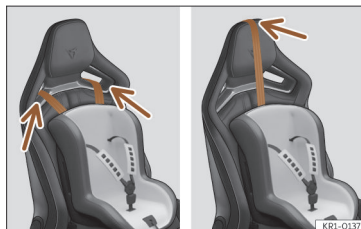
Abb. 43 Beifahrersitz: Einstellung und Einbau unter Verwendung des Top Tether-Gurts.
