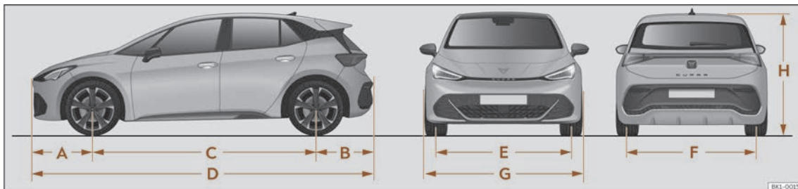
Abb. 171 Abmessungen
