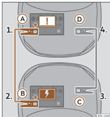
Abb. 148 Anschlussplan der Starthilfekabel.
